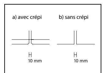
Système de joint ouvert
